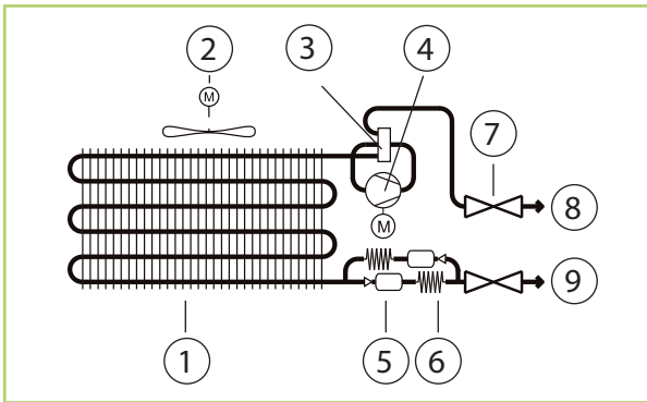
Obr. 10: Schéma zapojení okruhu chlazení vnější jednotky
