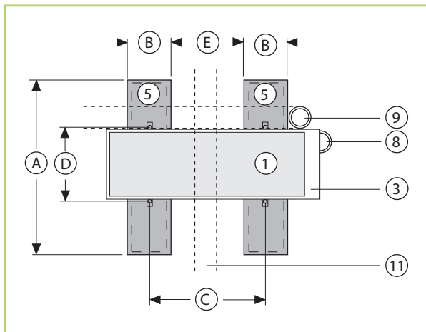
Obr. 39: Rozměrový výkres podezdívky (pohled shora)
