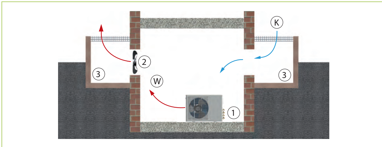
Obr. 28: Instalace uvnitř budovy
