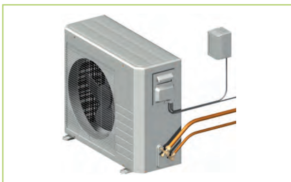
Obr. 42: Připojení vnější jednotky
