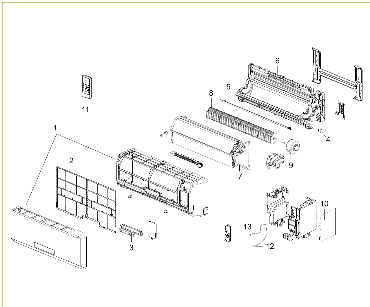
Obr. 52: Znázornění zařízení ML 263 DC IT-523 DC IT
