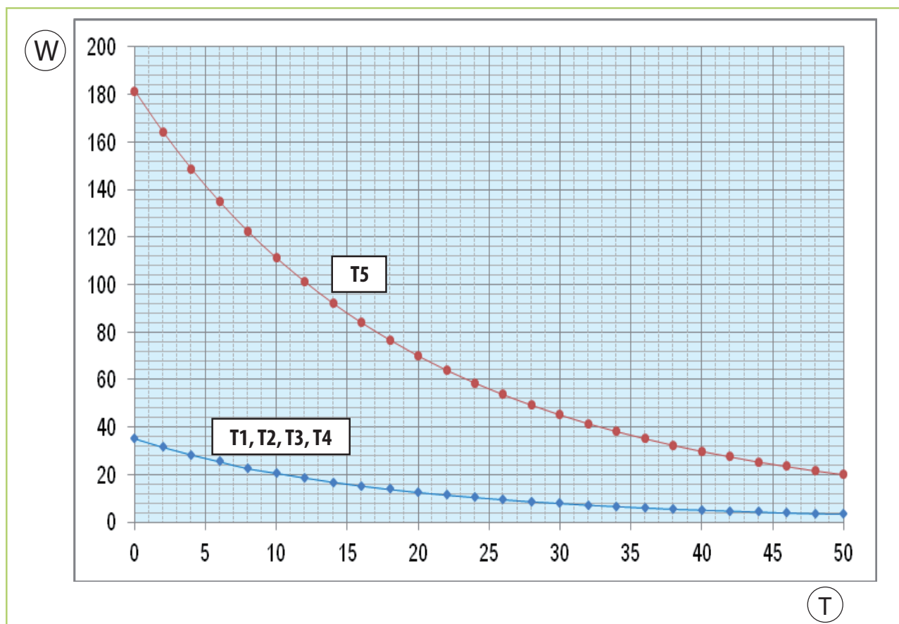
Obr. 48: Průběh teploty / odpor
