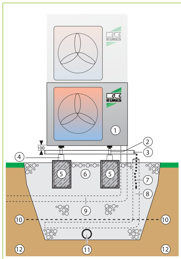
Obr. 38: Odvod kondenzátu, odvod kondenzátu do podezdívky (řez)
