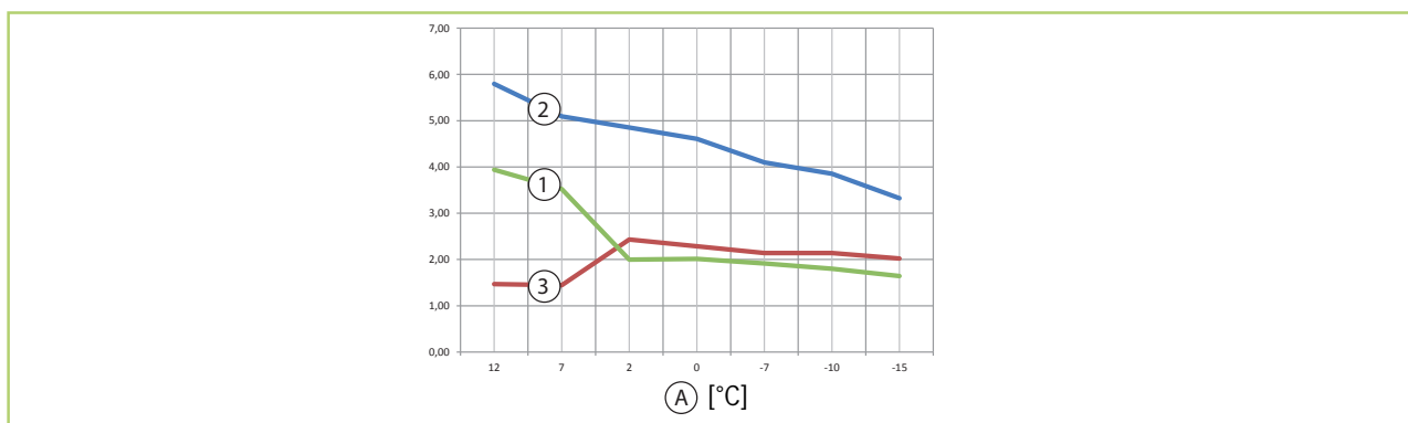
Obr. 7: Grafy výkonu topení ML 523 DC (údaje při vnitřní teplotě 20 °C)
