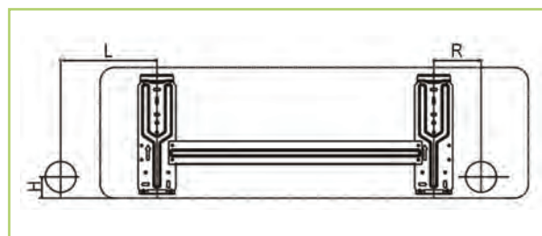
Obr. 32: Montážní body nástěnného držáku ML 263 DC IT-523 DC IT (čelní pohled, všechny rozměry v mm)
