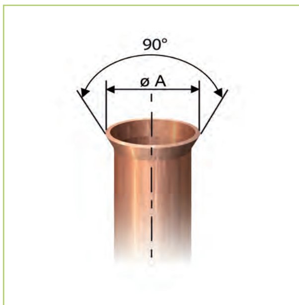
Obr. 36: Správný tvar flérování
