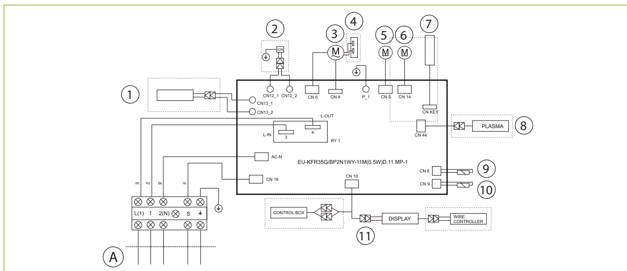
Obr. 44: Elektrické schéma zapojení
