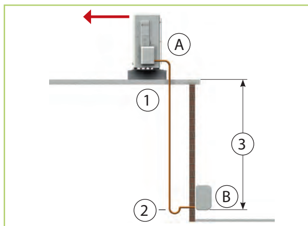
Obr. 30: Opatření pro zpětné vedení oleje
