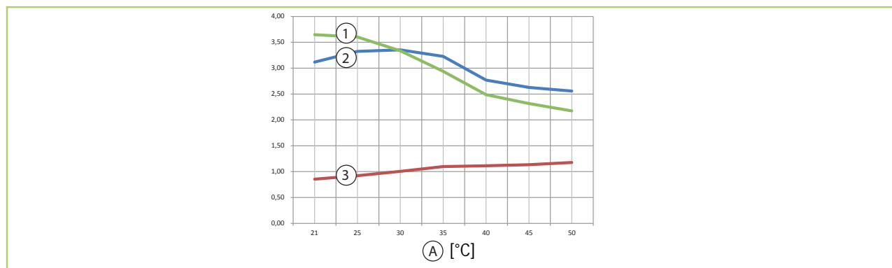
Obr. 6: Grafy výkonu chlazení ML 353 DC (údaje při vnitřní teplotě 27/19 °C)
