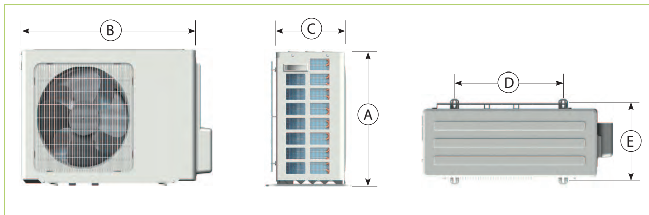
Obr. 1: Rozměry vnější jednotky ML 263 DC AT-523 DC AT (všechny údaje v mm)
