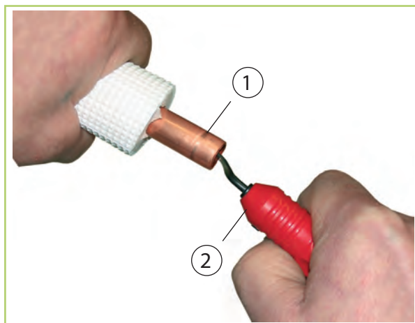
Obr. 34: Odhrotování vedení chladiva
