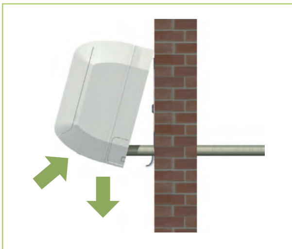
Obr. 33: Vodorovné vyrovnaní
