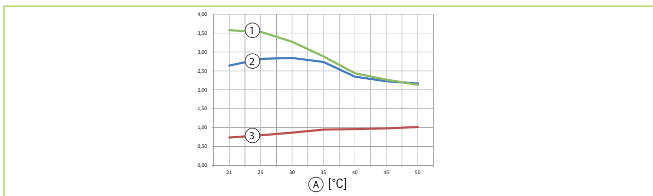
Obr. 4: Grafy výkonu chlazení ML 263 DC (údaje při vnitřní teplotě 27/19 °C)
