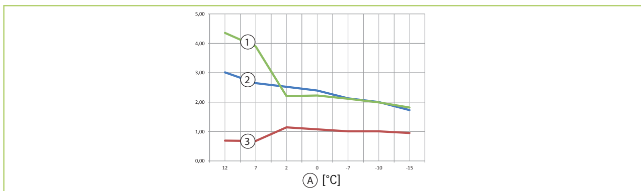
Obr. 3: Grafy výkonu topení ML 263 DC (údaje při vnitřní teplotě 20 °C)
