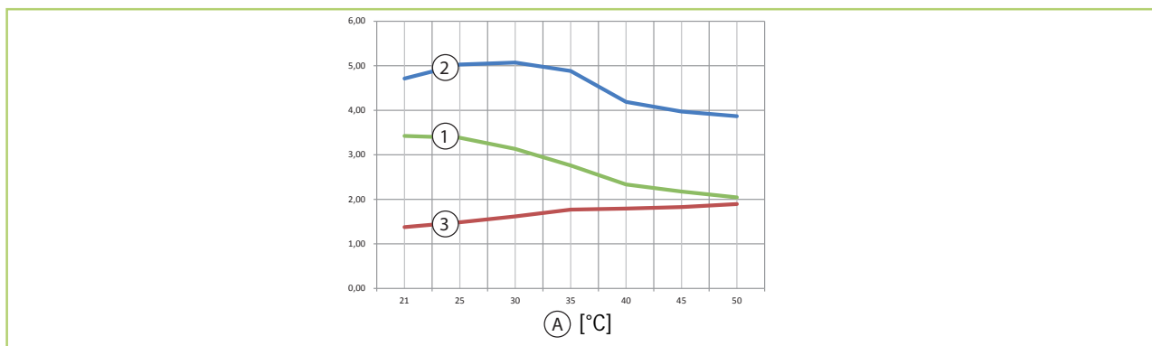
Obr. 8: Grafy výkonu chlazení ML 523 DC (údaje při vnitřní teplotě 27/19 °C)
