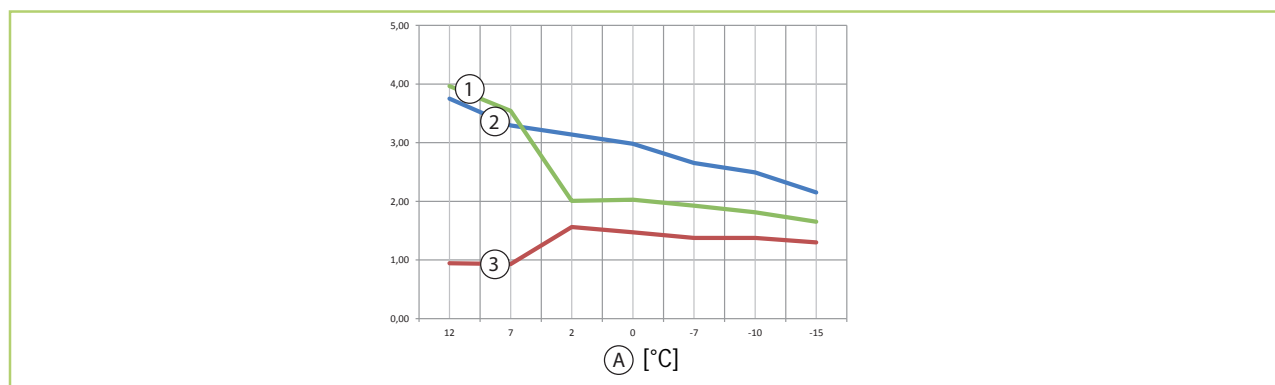
Obr. 5: Grafy výkonu topení ML 353 DC (údaje při vnitřní teplotě 20 °C)
