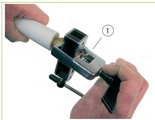
Obr. 35: Flérování vedení chladiva
