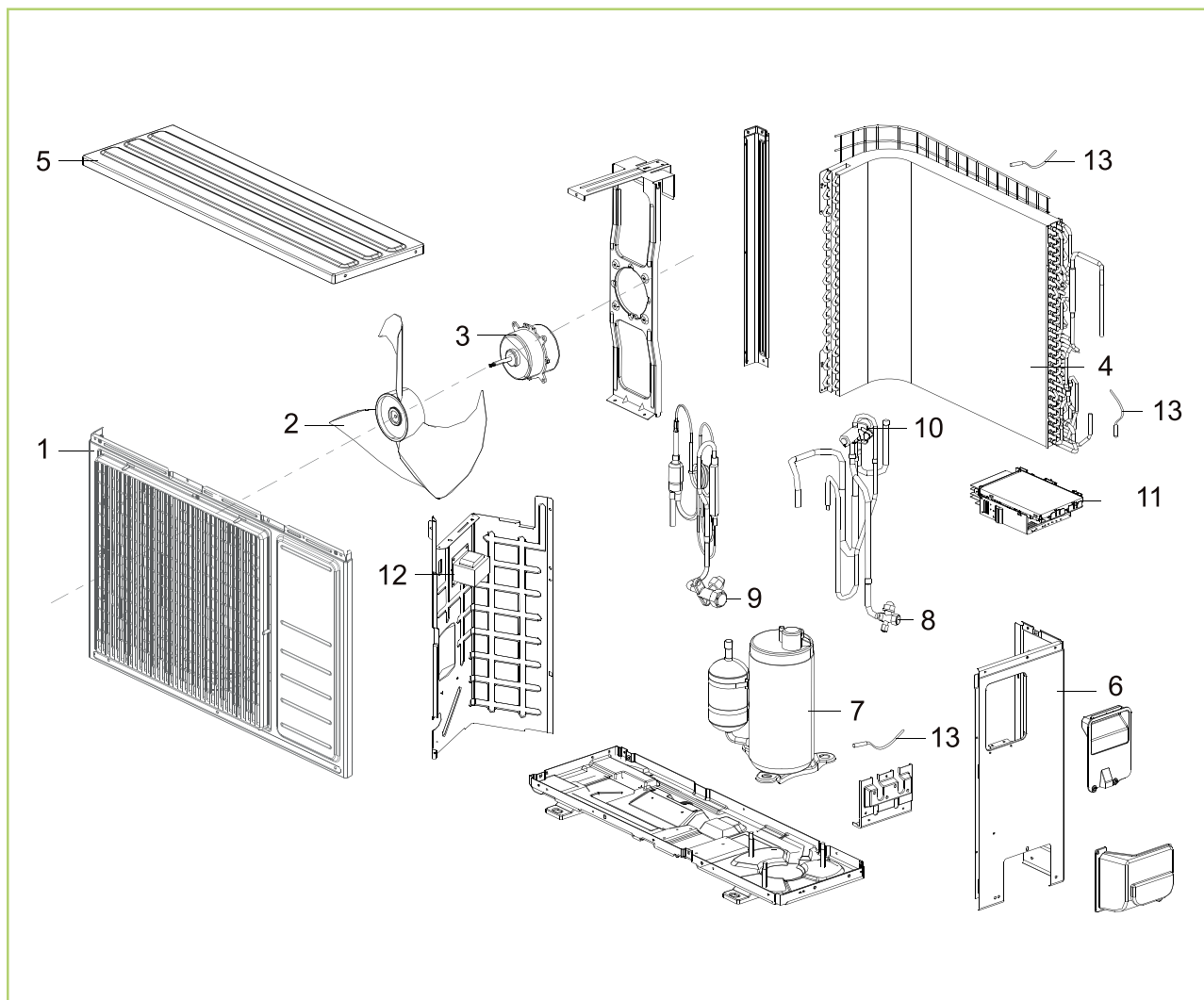
Obr. 53: Znázornění zařízení ML 263 DC AT-523 DC AT
