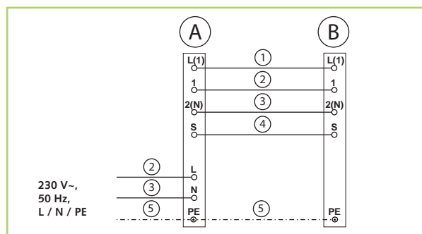
Obr. 43: Elektrické schéma připojení
