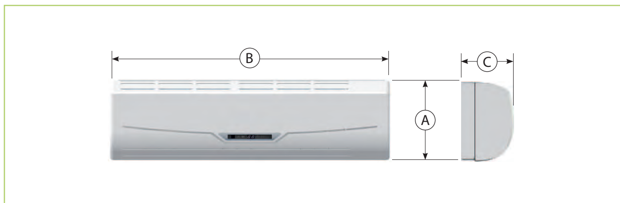
Obr. 2: Rozměry vnitřní jednotky ML 263 DC IT-523 DC IT (všechny údaje v mm)
