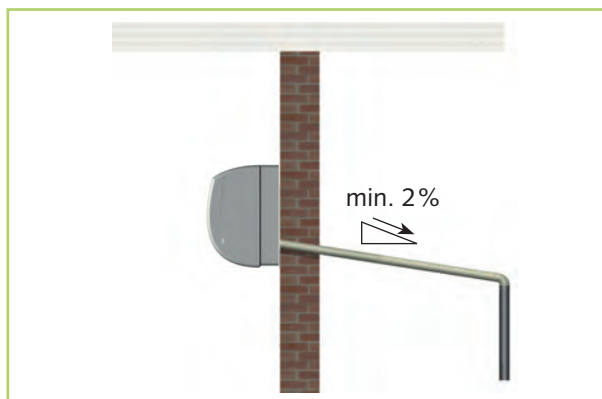
Obr. 40: Přípojka pro odvod kondenzátu vnitřní jednotky
