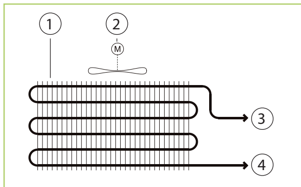
Obr. 9: Schéma zapojení okruhu chlazení vnitřní jednotky
