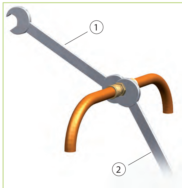
Obr. 37: Utažení šroubení
