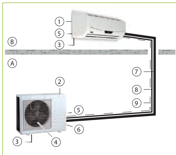
Obr. 11: Konstrukce systému
